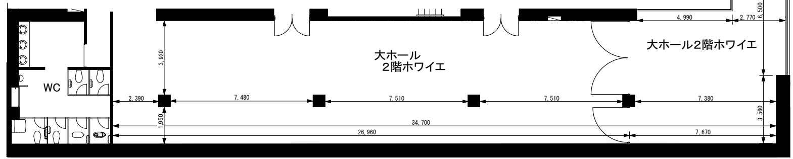
ホワイエ周り寸法 S=1/200
