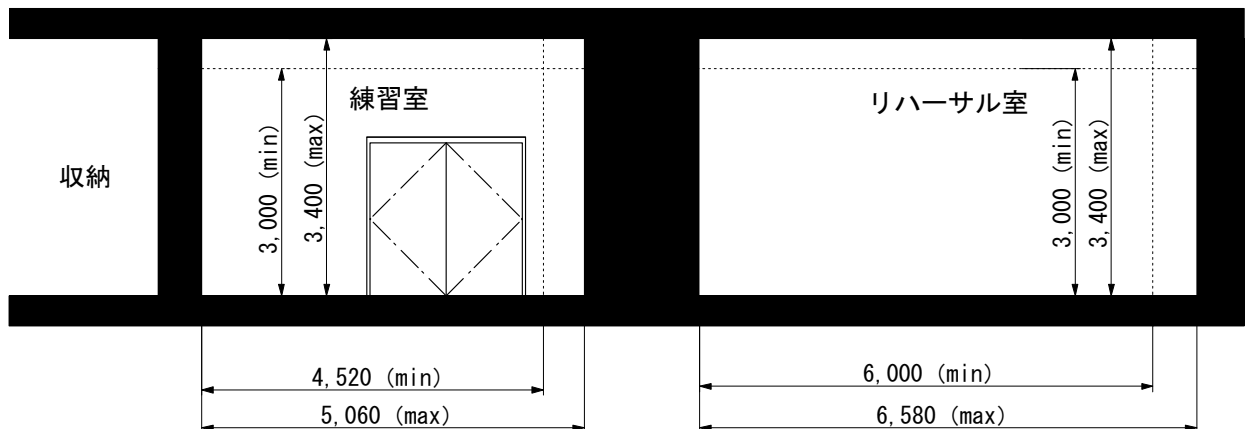
断面図 S=1/100
