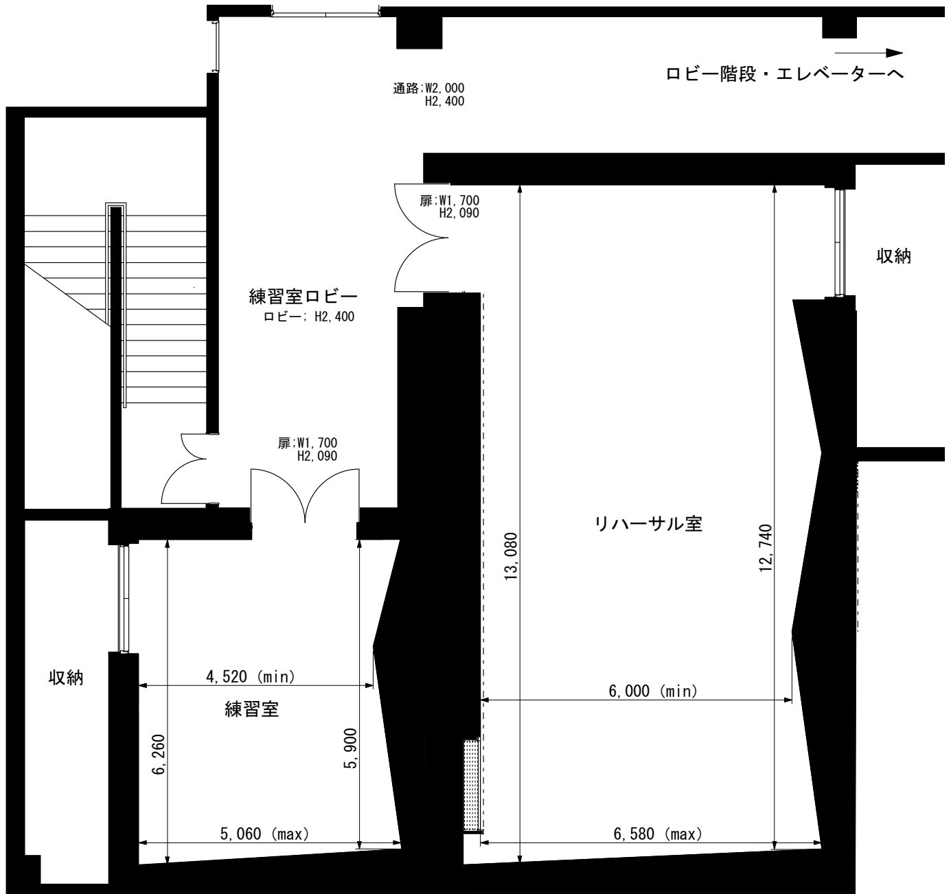
平面図 S=1/100
